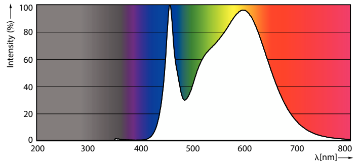
Spectral Power Distribution Colour - 14A19/CNG/840/FR/P/E26/D 12/1CT
