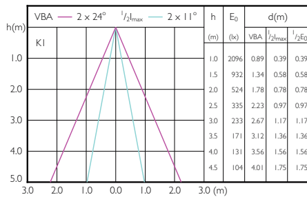
LEDSpots MR16 7W 930 430lm 25D
