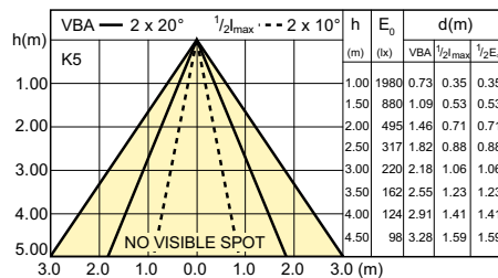
SDBE_LEDspotL_0127-Beam diagram
