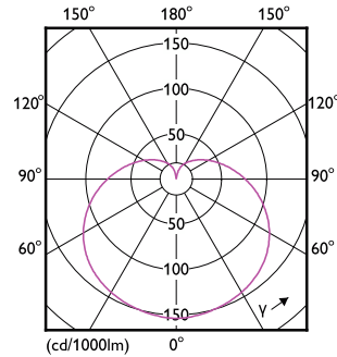
Light Distribution Diagram - 5A19/CNG/827/FR/P/E26/D 12/1CT
