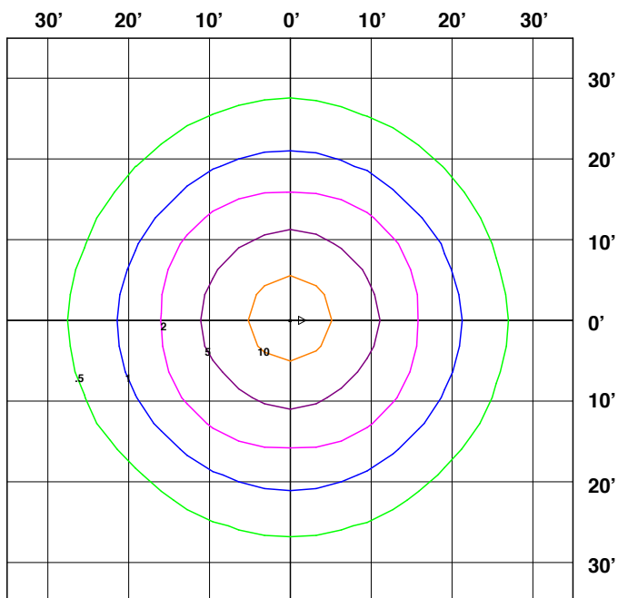
55W CANOPY 15'
