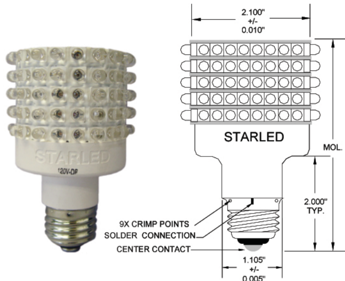
MODEL: EBWL205
