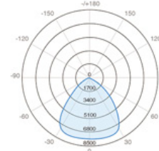
90° Reflector
