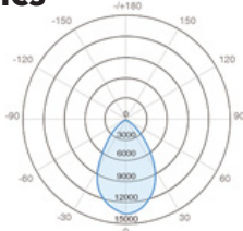
60° Reflector
