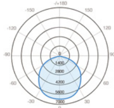
120°, Standard/no Reflector
