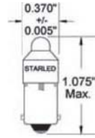
Miniature Bayonet 111
